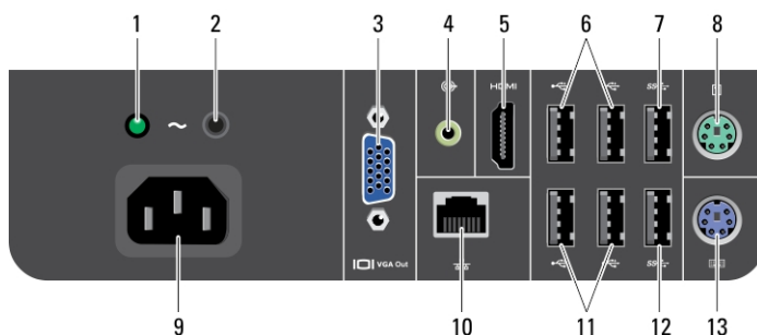
图 3: 背面板视图
